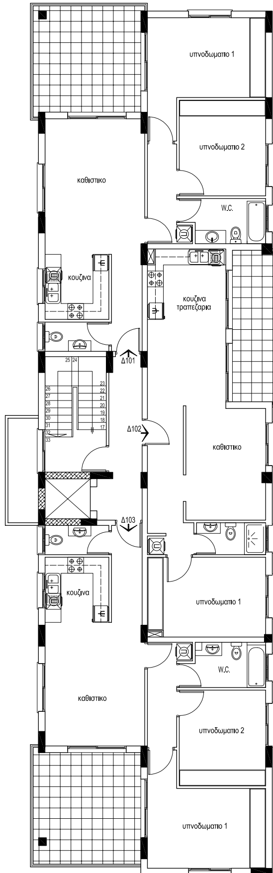
κατοψη 1ου οροφου κλ. 1 : 100
