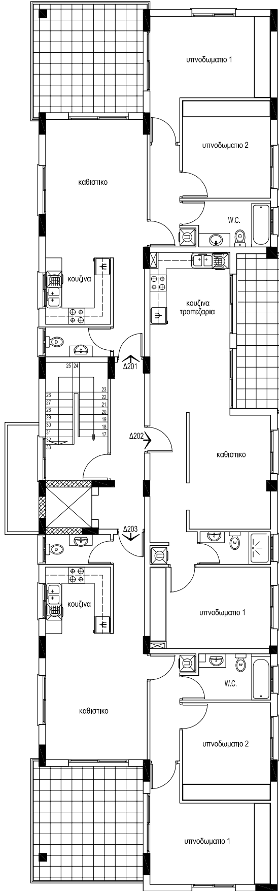
κατοψη 2ου οροφου κλ. 1 : 100
